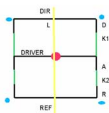
YU1QTs 3 elements Moxon för 40.
